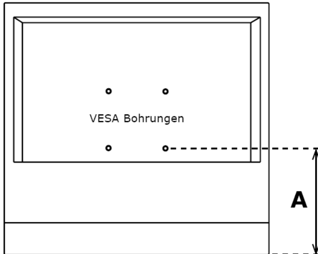
Rückansicht TFT-Monitor
