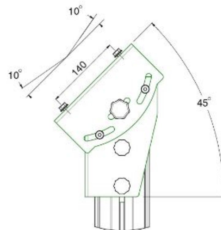
DETAIL B SCALE 0.150
